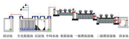
清洁池 生化脱氮池 沉淀池 中间水池 表面湿地 一级潜流湿地 二级潜流湿地 清水池
